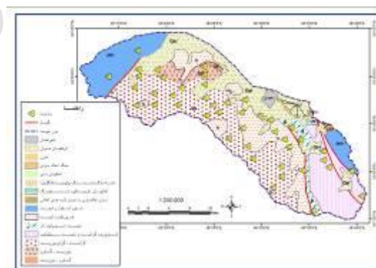
شکل ۴. موقعیت واریزه‌ها در دامنه‌های شمالی الوند
