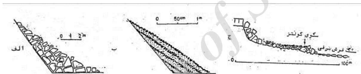
شکل ۱. انواع مختلف جریان واریزه‌های الف) جریان واریزه ثقلی ب) واریزه‌های لایه‌لایه
