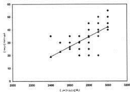
نمودار ۱. رابطه همبستگی شیب دامنه با ارتفاع واریزه‌ها
