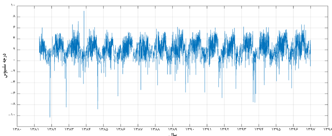
شکل ۵. شدت جزیره گرمایی / سرمایی شهر اهواز، آکوا گذر شب (منبع: نویسندگان، ۱۳۹۷)
