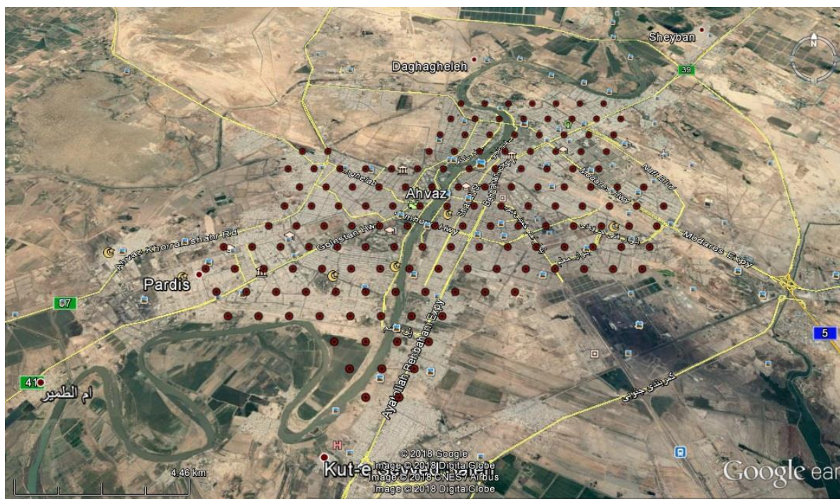
شکل ۱. یاخته‌های مودیس درون مرز شهر اهواز (منبع: نویسندگان، ۱۳۹۷)
