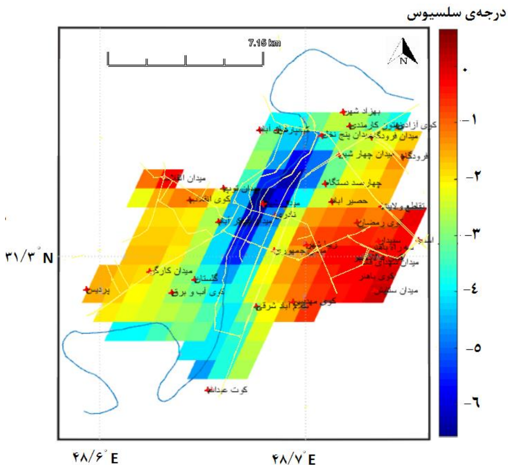
شکل ۷. میانگین بلندمدت جزیره گرمایی اهواز؛ آکوا، روز (منبع: نویسندگان، ۱۳۹۷)
