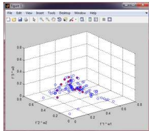
شکل ۱۰. نمایش تنوع در جوابهای پیشنهادی غیرمسلط بهینه پرتو با بردارهای وزن تصادفی و نمایش پرتو فرونتها (نقاط قرمز رنگ)
