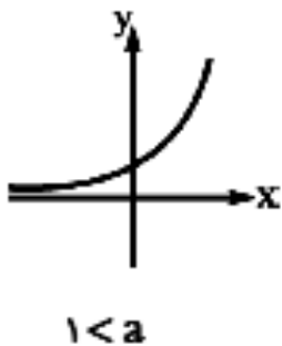
شکل ۳۲. نمودار تابع‌نمایی (۲)
