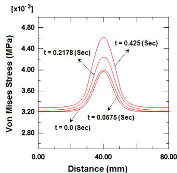
شکل (۶): نمودار تنش ون‌میزز بر روی سطح بالایی مدل بافت شامل شریان در چهار زمان متفاوت از مرحله سیستمولیک (۱۰).
