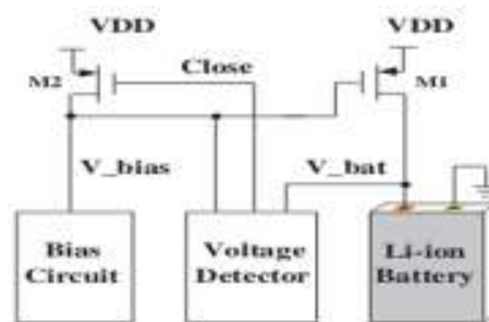
شکل ۸: بلوک دیاگرام شارژ باتری
