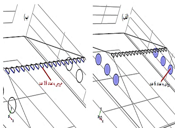
شکل ۱۹. (الف) ورودی جریان هوا به تعداد ۶ دریچه از کنار سقف شیروانی و (ب) خروجی جریان هوا به تعداد ۱۸ دریچه از روی سقف شیروانی.
