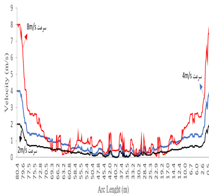
شکل ۲۲. مقایسه منحنی تغییرات سرعت ورودی هوا برحسب طول شیروانی به ازای سرعت‌های ۲ m/s، خط سیاه، ۴ m/s، خط آبی و ۸ m/s، خط قرمز.
