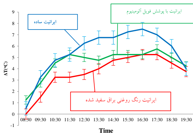
شکل ۹. میانگین تفاوت دمای اتاقک با بیرون برای اتاقک با ایرانیت ساده، خط آبی، با ایرانیت با پوشش برگه آلومینیوم، خط سبز، و با ایرانیت رنگ شده سفید براق، خط قرمز، برحسب ساعت روز. میانگین دمای ۷ الی ۹ شهریور ۱۳۹۸ است.
