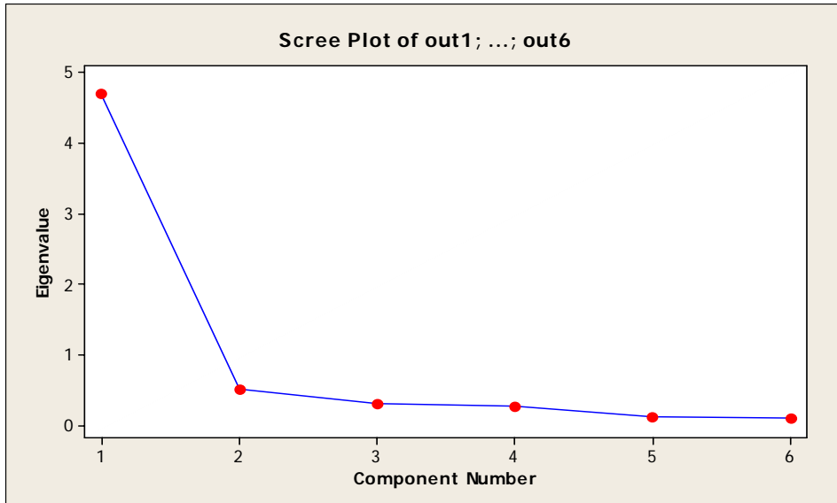
نمودار ۱. نمودار سنگریزه مؤلفه‌های اصلی
