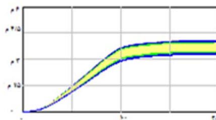
شکل ۲۴. تأثیر تغییر هزینه تعمیرات و نگهداری بر تجمعی الکتریسته تولیدی توسط فناوری
