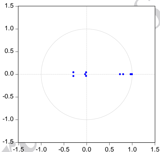
نمودار ۱. بررسی ریشه‌های مشخصه مدل VAR
