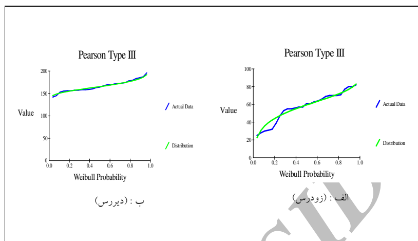
شکل (۲) برازش داده‌ها روی توزیع پیرسون تپ ۳
