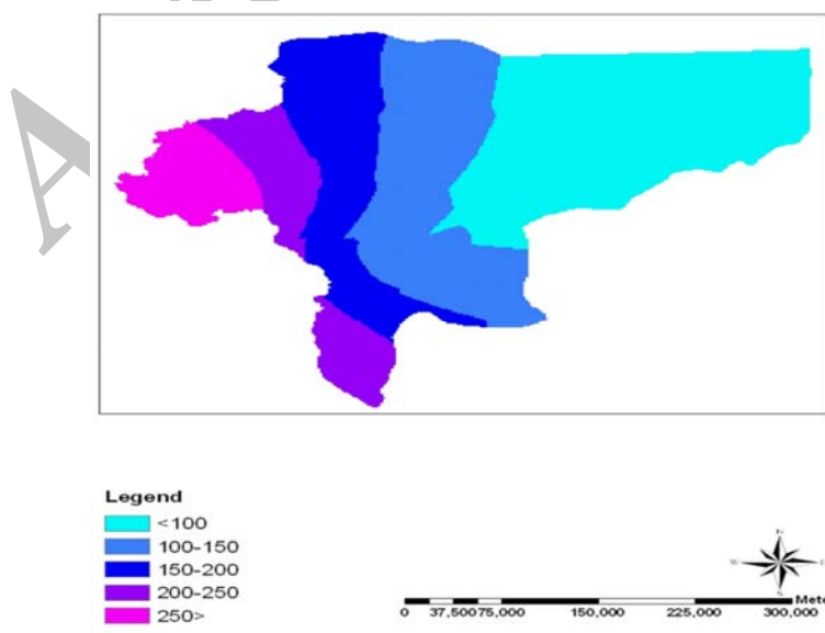
شکل شماره 11- نقشه همبارش استان اصفهان به روش Kriging
