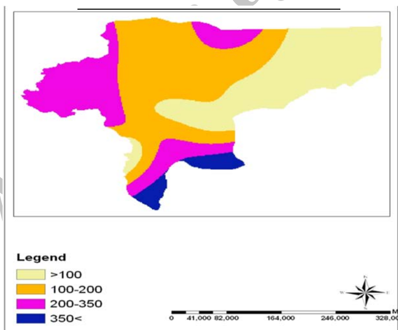
شکل شماره 12- نقشه همبستگی بارش استان اصفهان به روش همبستگی بارش و طول جغرافیایی
