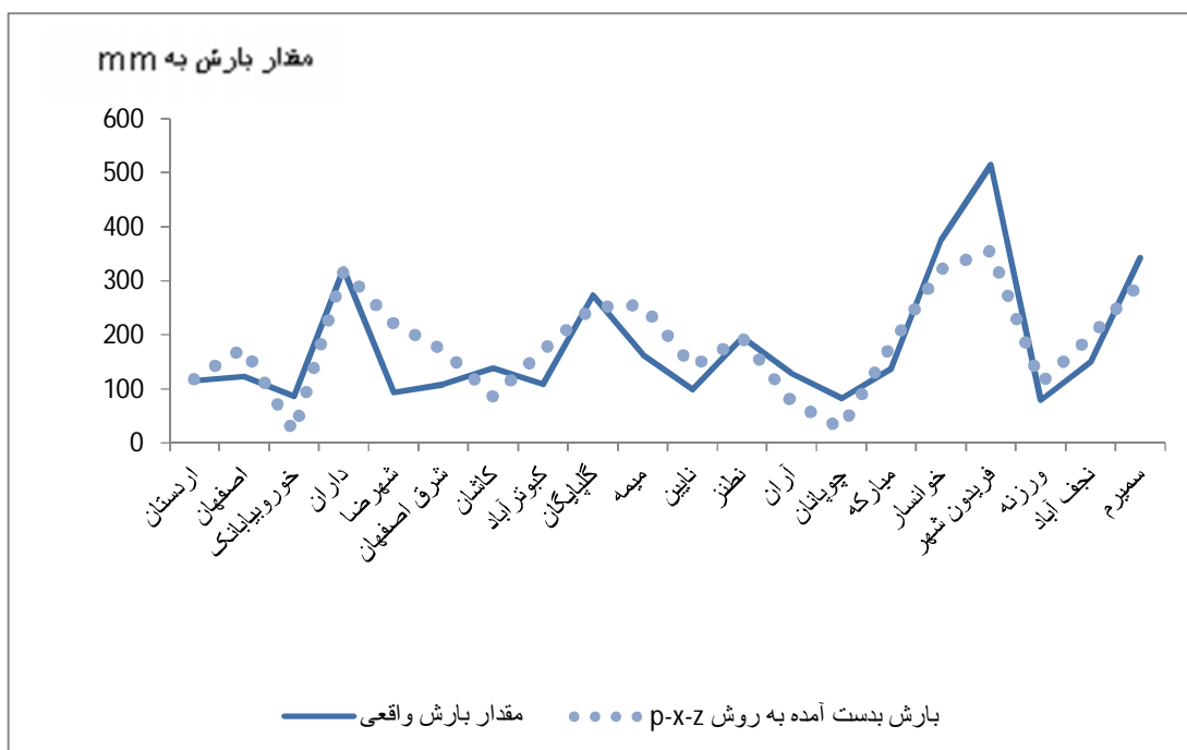
شکل شماره 5- نمودار مقایسه بارش واقعی و بارش به دست آمده به روش اقلیمی (بارش و طول جغرافیایی و ارتفاع z-x-p)
