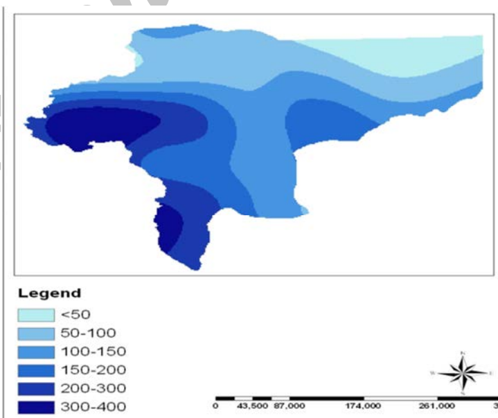
شکل شماره 14- نقشه همبارش استان اصفهان به روش همبستگی بارش، ارتفاع و طول جغرافیایی
