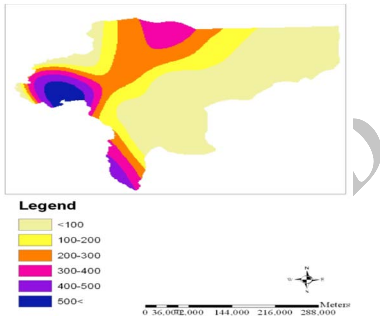
شکل شماره 10: نقشه همبارش استان اصفهان به روش Spiline
