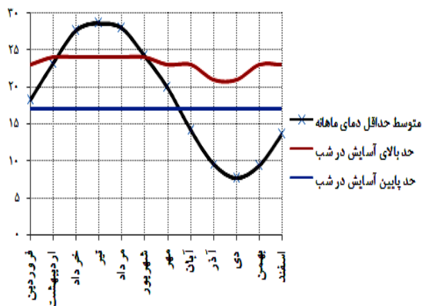
نمودار ۵- مقایسه متوسط دمای هوای در روزهای ماه‌های
