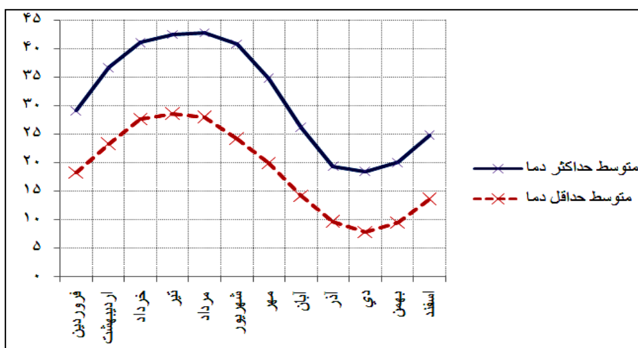
نمودار ۱- تغییرات ماهانه متوسط حداکثر و متوسط حداقل دمای هوا در خرمشهر
