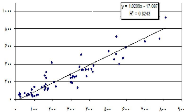
دبی رسوب محاسباتی ( میلی گرم در لیتر)
