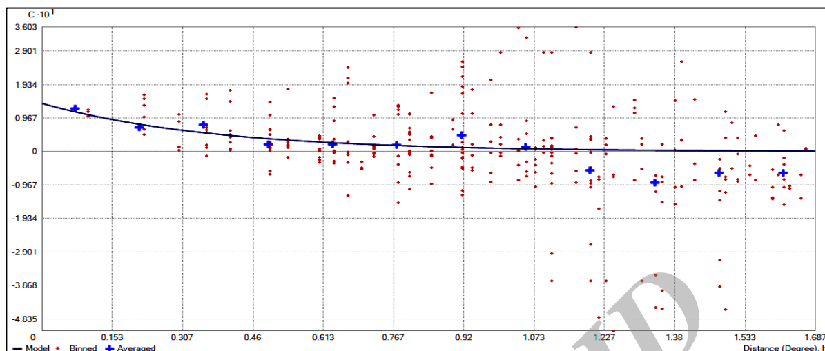
شکل ۵: منحنی نیم تغییرنمای متقابل محاسبه شده‌ی روش کوکریجینگ با مدل تنورکی برازش داده شده به آن
