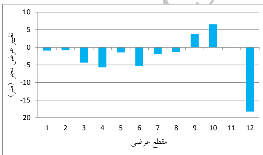
شکل ۹: تغییرات عرض مجرا رودخانه ليقوان چای در دوره مورد مطالعه
