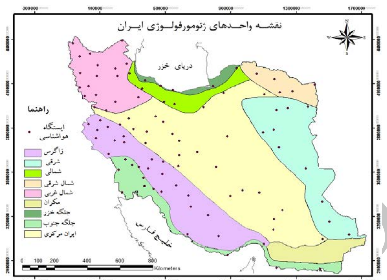
شکل ۱: حدود تقریبی واحدهای ژئومورفولوژی ایران
