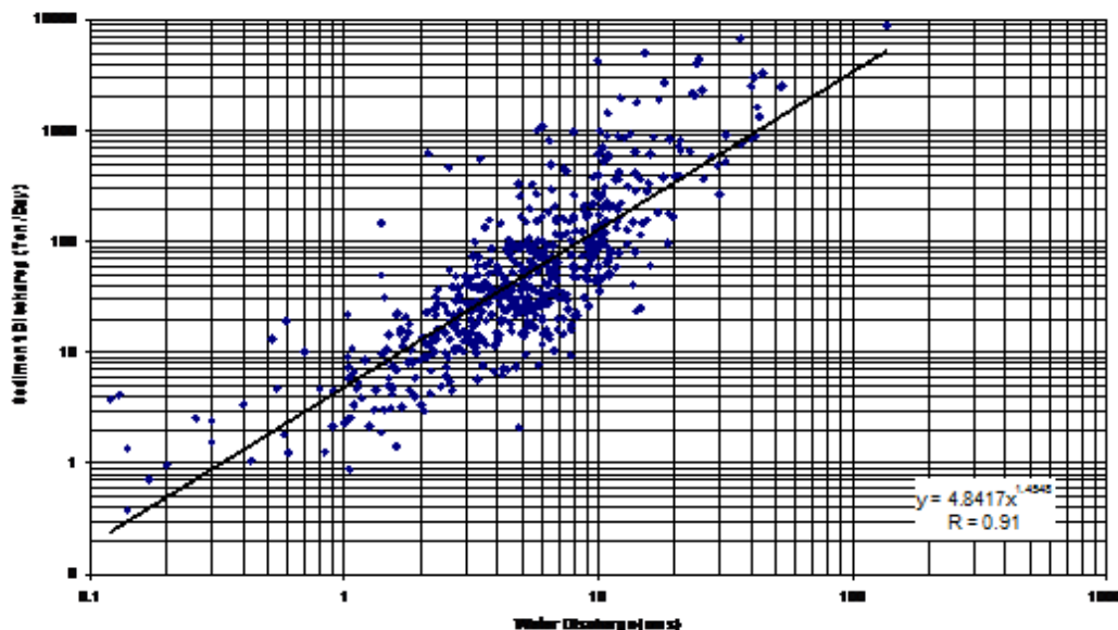
شکل ۴: منحنی سنجه رسوب حوضه آبریز بابلرود (AILWMP، 2008)
