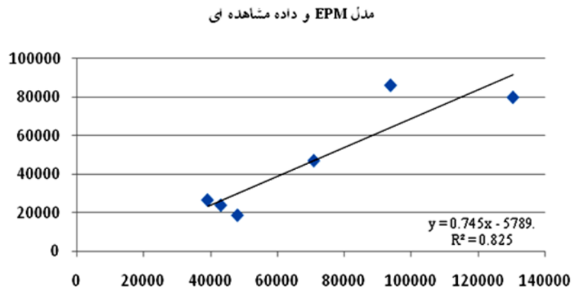
شکل ۳: نمودار همبستگی بین نتایج مدل EPM و داده‌های مشاهده‌ای
