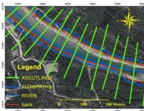
شکل ۱۰: نمایی از نقشه رقومی زمین و مقاطع عرضی
