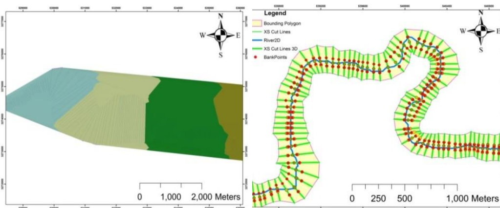
شکل ۱۱: نمای داده‌های ورودی به الحاقیه Hec-GeoRAS شکل ۱۲: نمایی از سطح محدوده‌ی مطالعاتی در الحاقیه HEC-GeoRAS
