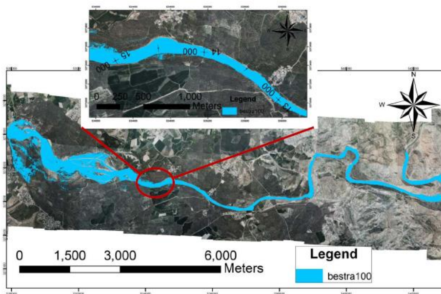
شکل ۱۸: پهنه‌ی سیلاب رودخانه‌ی شاپورخشت با دوره بازگشت ۱۰۰ سال
