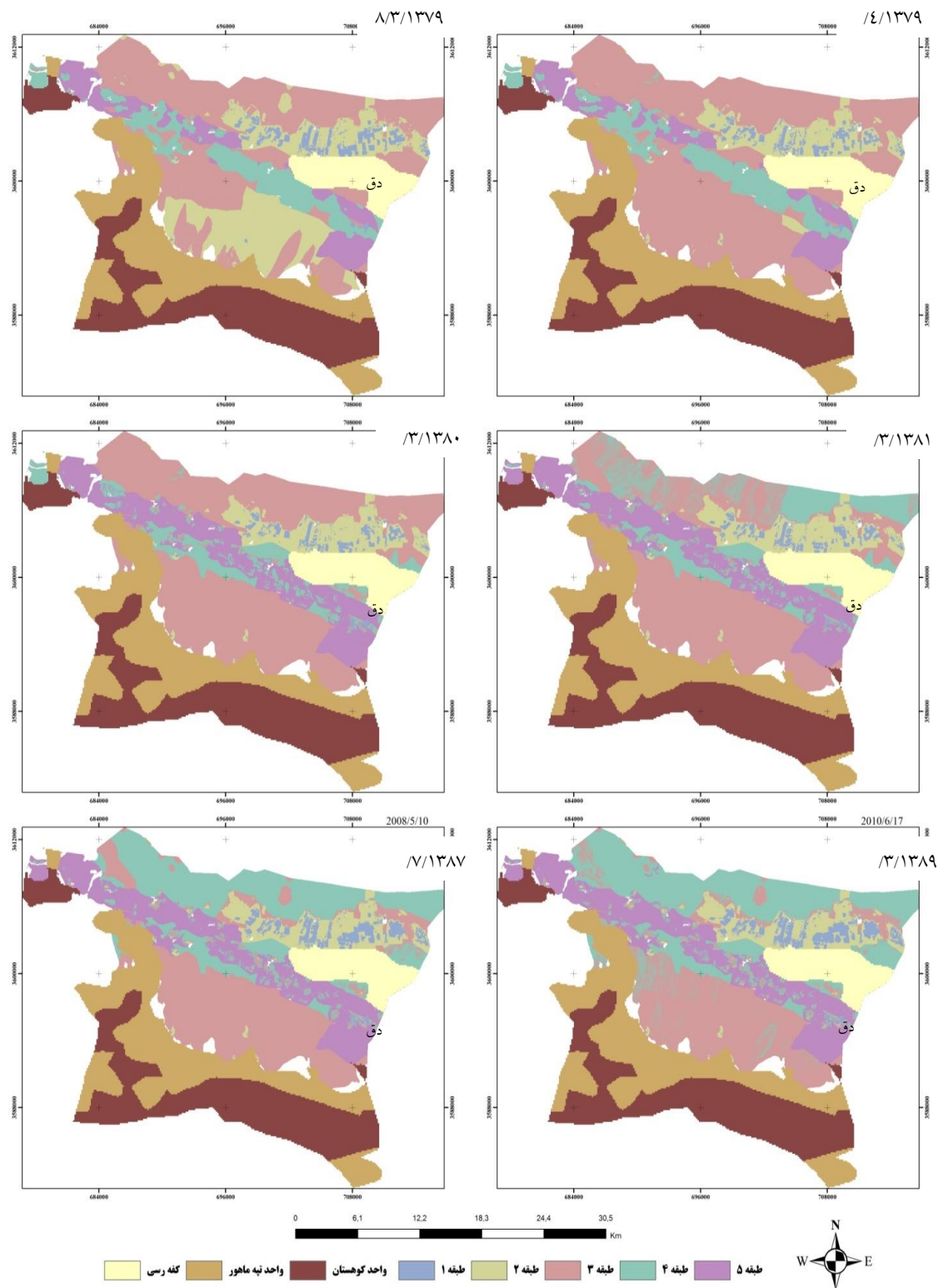
شکل ۶: تغییرات پهنه‌های فرسایش بادی در دوره‌های مورد بررسی حاصل از در نظر گرفتن تغییرات زمانی و مکانی کاربری و پوشش زمین
