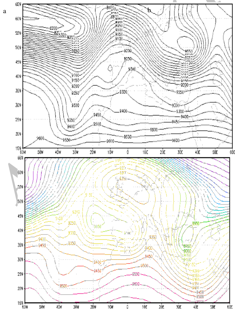
شکل ۱۲: ارتفاع ژئوپتانسیل تراز ۳۰۰ هکتوپاسکال = فاز منفی و = فاز مثبت
