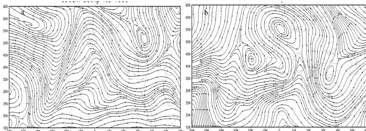
شکل ۱۴: جریان هوا در تراز ۵۰۰ هکتوپاسکال = فاز منفی و b = فاز مثبت
