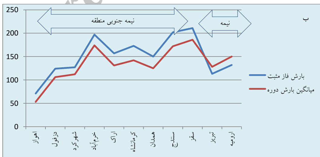
شکل ۱۱: تفاوت بارش میانگین (MM) فصل بهار و مقایسه آن‌ها با میانگین بارش دوره آماری الف. فاز منفی ب. فاز مثبت
