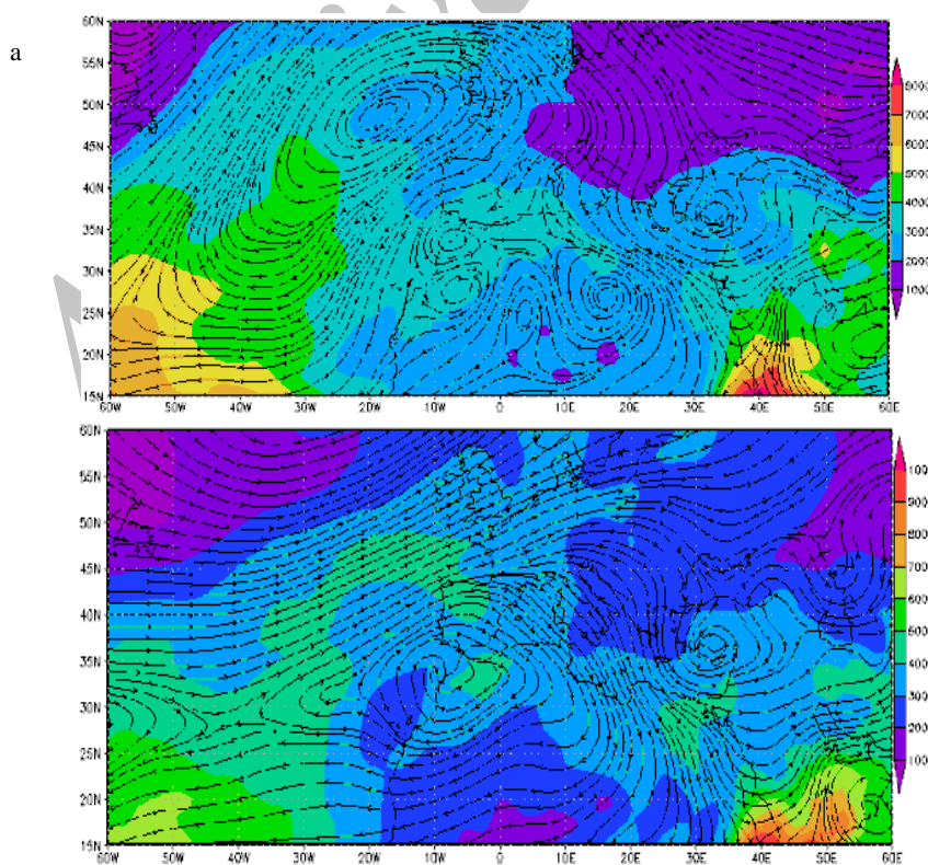
شکل ۱۵: وزش رطوبت در تراز ۸۵۰ هکتوپاسکال = فاز منفی و b = فاز مثبت
