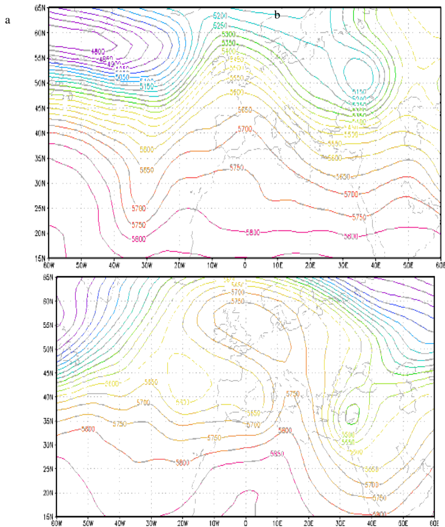
شکل ۱۳: ارتفاع ژئوپتانسیل تراز ۵۰۰ هکتوپاسکال =a فاز منفی و b = فاز مثبت
