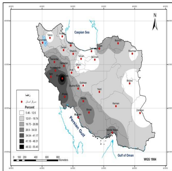
شکل ۲: طیف سنجی درصد فراوانی آرای کروی
