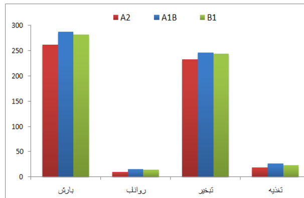
شکل ۴: مقادیر میانگین سالانه بارش، رواناب، تغذیه آب زیرزمینی و تبخیر و تعرق تحت سناریوهای A2، B1 و A1B برای دوره (۲۰۳۰-۲۰۱۳) در حوضه آبریز تسوج
