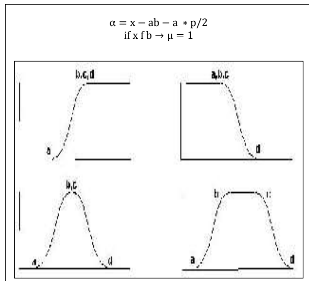
شکل ۳: تابع Sigmoidal
