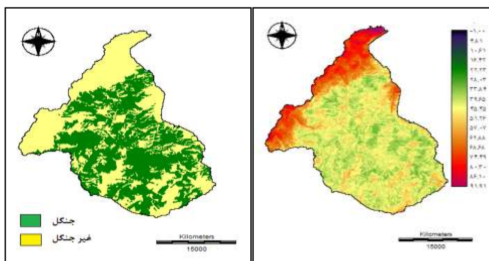
شکل ۷: نقشه‌های تناسب و پیش‌بینی شده پوشش جنگلی حاصل از مدل ژنومد
