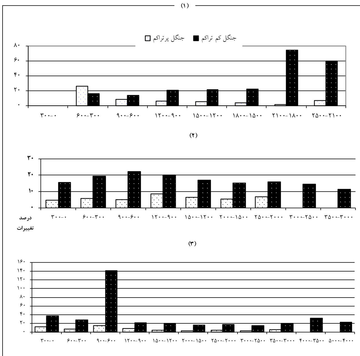
شکل ۴: درصد تغییرات (محور عمودی) هر یک از کلاسه ها نسبت به سطح اولیه در سال (۱۳۶۹) در هر یک از طبقات متغیرهای ارتفاع به متر (۱)، فاصله از جاده به متر (۲)، فاصله از مسکونی به متر (۳)، طبقات جهت (۴)، طبقات شیب به درصد (۵)
