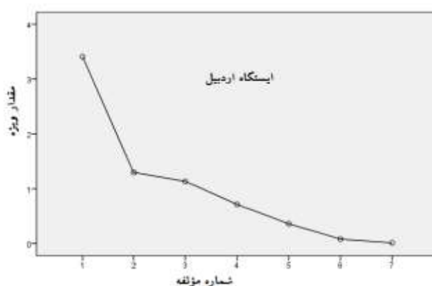
شکل ۳: نمودار واریزه‌ای (Scree Plot) در ایستگاه اردبیل
