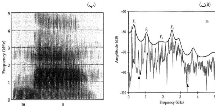
شکل ۲: طیف FFT، LPC و طیف‌نگاشت کلمهٔ تایلندی [ma] (برگرفته از جانسون، ۲۰۰۳: ۱۵۸)
