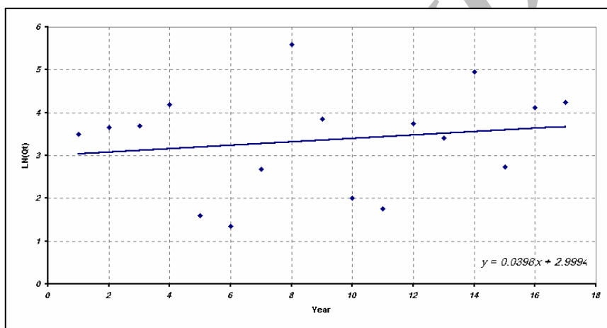
شکل (۵) نمودار LN Trend (TS) در دوره آماری ۱۳۸۰-۱۳۷۹ تا ۱۳۶۴-۱۳۶۳
