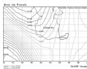
شکل ۱۴ نقشه نمایان سطح متوسط دریا بهاره گرگانرود در دوره قبل از وقوع سیل
