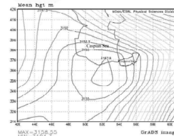
شکل ۱۴ نقشه ارتفاع متوسطه-۱۰ فکوناسکال بعد از جبهه گرگانه در دوره قبل از وقوع سیل
