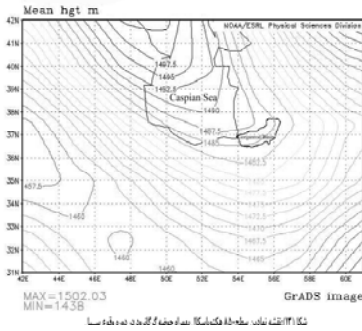
شکل ۱۱ نقشه ارتفاع متوسطه-بالا فکوناسکال بعد از جبهه گرگانه در دهه ۱۹۵۰
