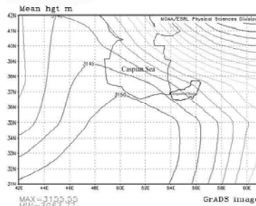
شکل ۱۳ نقشه ارتفاع متوسطه-۱۰ فکوناسکال بعد از جبهه گرگانه در دوره وقوع سیل
