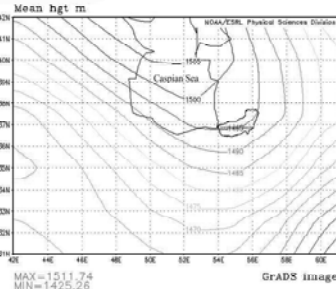
شکل ۱۲ نقشه ارتفاع متوسطه-بالا فکوناسکال بعد از جبهه گرگانه در دوره قبل از وقوع سیل
