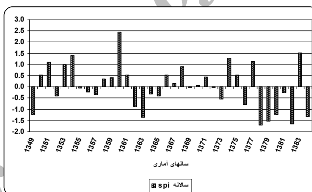
شکل شماره ۵: نمودار تغییرات SPI بارش سالیانه ایستگاه کليماتولوژی بمپور طی دوره مورد مطالعه
