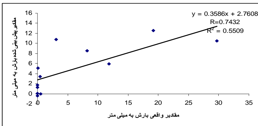
شکل شماره (۱۵) پراکنش نگار و خط برازش یافته بین مقادیر واقعی ماهانه بارش و پیش بینی شده توسط شبکه در حالت تصادفی در ترکیب با الگوریتم ژنتیک
