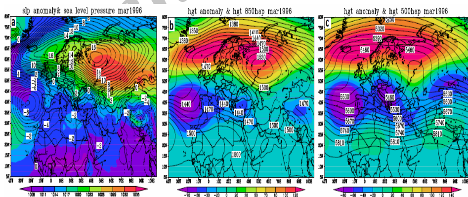
شکل (۹) میانگین و ناهنجاری فشار تراز دریا (a) و ارتفاع ژئوپتانسیل تراز ۸۵۰ (b) و ۵۰۰
