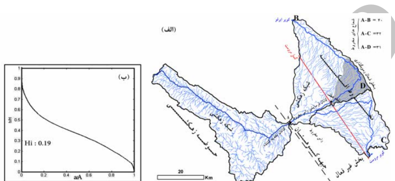
شکل (۲) ویژگی‌های فیزیوگرافی حوضه آبریز مروست (بوانات)
