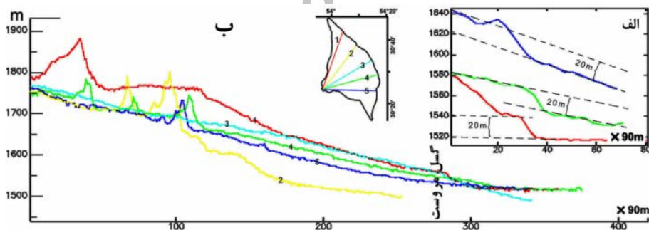
شکل (۴) پروفیل‌های عمود بر راستای گسل و (ب) پروفیل‌های شعاعی در مخروط‌افکنه مروست
