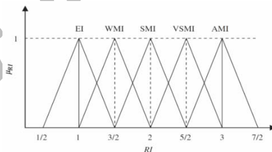
شکل (۱) مقیاس‌های زبانی برای بیان درجه اهمیت
