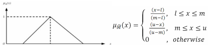
شکل (۲) عملکرد عضویت یک عدد فازی سه وجهی \tilde{M} = (l, m, u)
