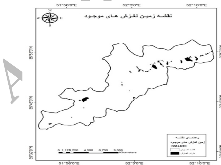
شکل (۳) پراکنش زمین لغزش های موجود در منطقه
