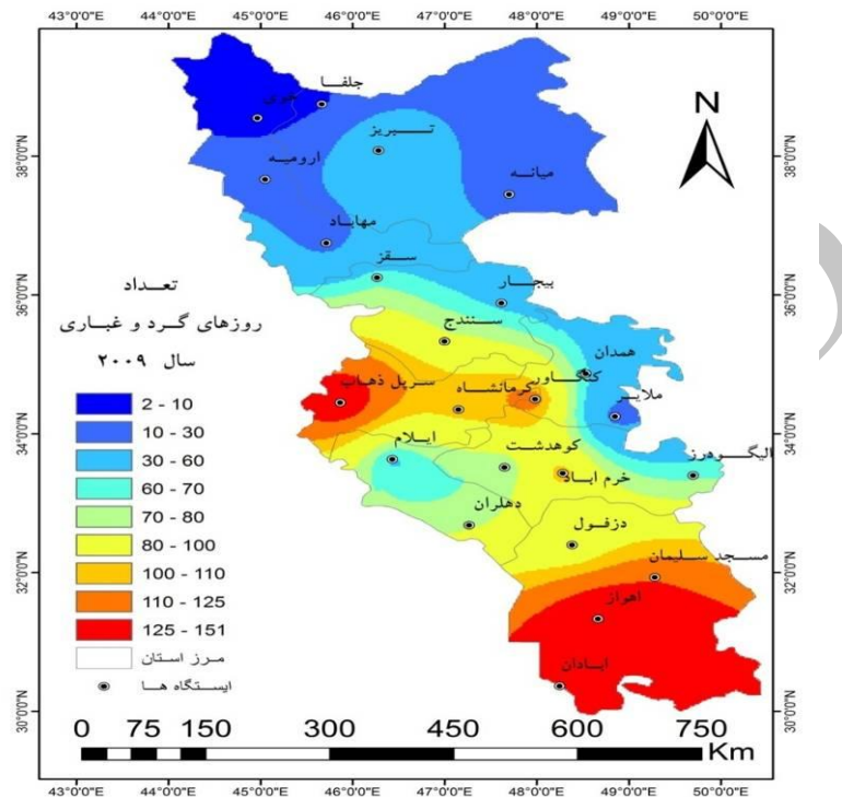
شکل (۴) پهنه بندی مجموع تعداد روزهای گرد و غباری در سال ۲۰۰۹
