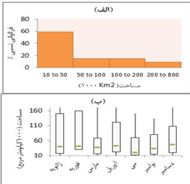
شکل (۹) الف: توزیع فراوانی مساحت MCS ب: نمودار جعبه‌ای مساحت MCS در هر ماه (۲۰۰۱-۲۰۰۵)
