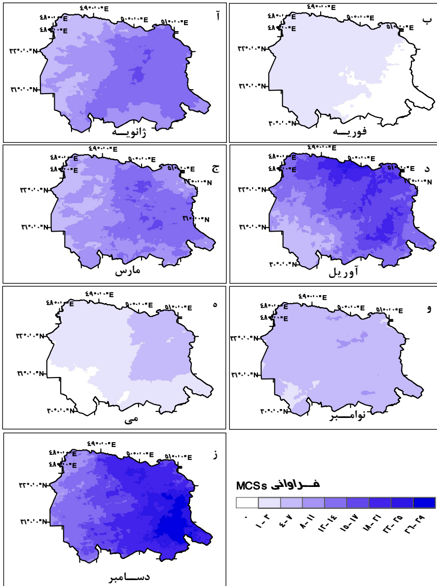
شکل (۷) پراکندگی مکانی رخداد سامانه‌های همرفتی میان‌مقیاس در جنوب غرب ایران (الف): زانویه؛ (ب): فوریه؛ (ج): مارس؛ (د): آوریل؛ (ه): می؛ (و): نوامبر؛ (ز): دسامبر
