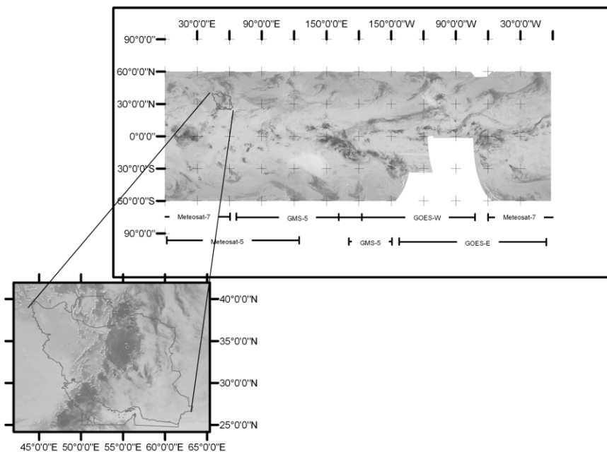
شکل (۳) تصویر دمای درخشندگی حاصل از باند مادون قرمز در روز ۱۷ آوریل ۲۰۰۵ ساعت ۰۲:۳۰ دقیقه
