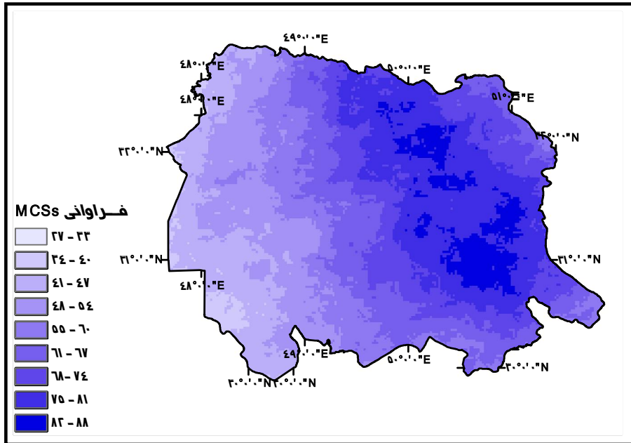
شکل (۸) پراکندگی مکانی رخداد سامانه‌های همرفتی میان‌مقیاس در جنوب غرب ایران (۲۰۰۱-۲۰۰۵)
