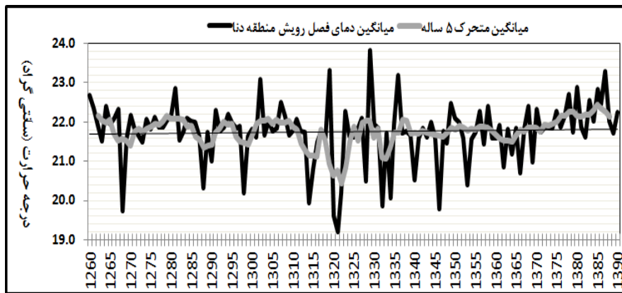
شکل (۷) مقدار میانگین دمای بازسازی شده اردیبهشت - شهریور، بر اساس گاه شناسی باقیمانده سه رویشگاه سی سخت، میمند و یاسوج جنگل های منطقه دنا در ارتفاعات زاگرس مرکزی ایران، طی یک دوره ۱۳۱ ساله (۱۳۹۰-۱۲۶۰)
