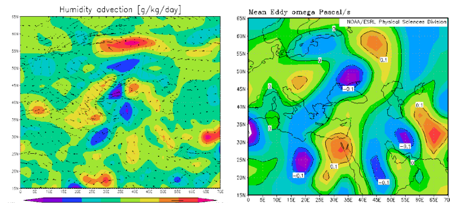
شکل (۱۶) نقشه پراکنندگی شاخص امگا در تراز ۷۰۰ hpa (راست) و وزش رطوبتی در تراز ۸۵۰ hpa (چپ) در روز نمونه الگوی پنجم (۳۰ آوریل ۱۹۷۶)
