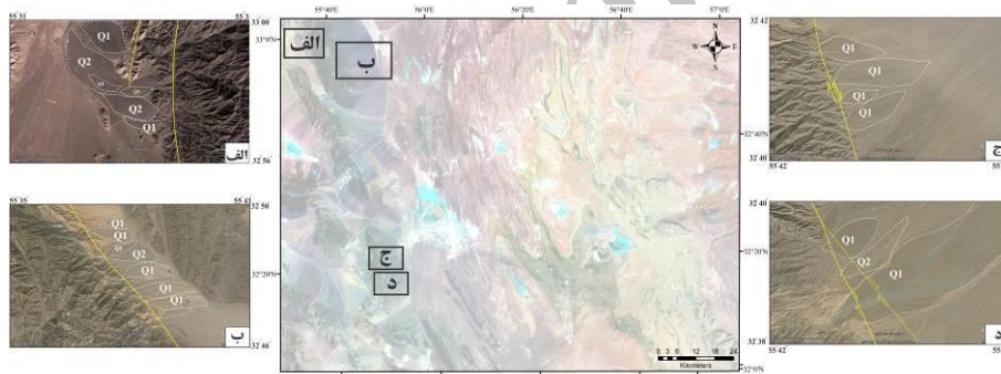
شکل ۱۰. مخروط افکنه‌های قدیمی (Q 1 ) و جدید (Q 2 ) (الف و د) نهشته شدن مخروط‌های جدید بر روی مخروط‌های قدیمی بر اثر فعالیت مجدد منطقه، (ب) جابجایی مخروط افکنه‌ها در اثر حرکت گسل (ج) حفر مجدد مخروط‌ها توسط آبراهه‌ها در اثر بالا آمدگی منطقه.
