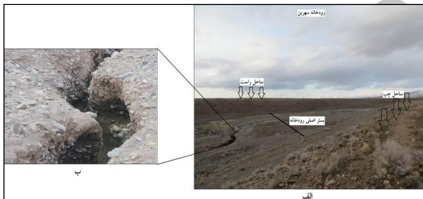
شکل (۵). بستر اصلی سهرین (الف) و عمیق کنی رودخانه (ب)
