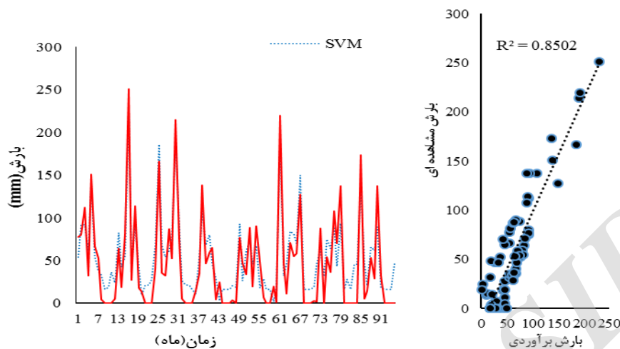
شکل (۲): مقادیر بارش مشاهده‌ای در برابر مقادیر برآوردی مدل SVM.
