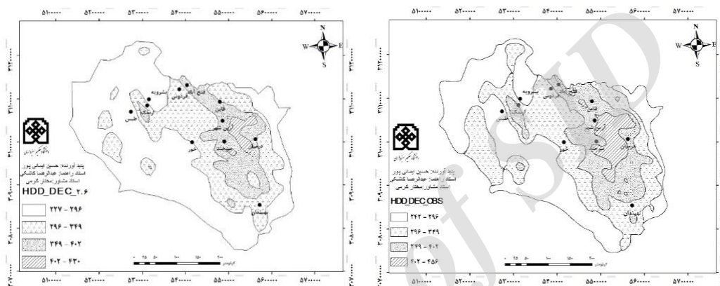
شکل (۱۴). پراکنش مکانی نیازهای گرمایشی آذر در دوره مشاهده ای (۱۹۹۰-۲۰۱۵) شکل (۱۵). پراکنش مکانی نیازهای گرمایشی آذر در دوره
