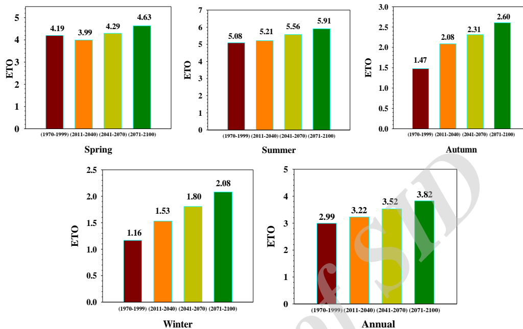
شکل (۶). میانگین سالانه و فصلی تبخیر و تعرق مرجع در دوره‌های مختلف تحت سناریوی RCP8.5 در ایستگاه
