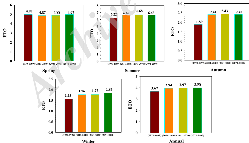
شکل (۷). میانگین سالانه و فصلی تبخیر و تعرق مرجع در دوره‌های مختلف تحت سناریوی RCP2.6 در ایستگاه
