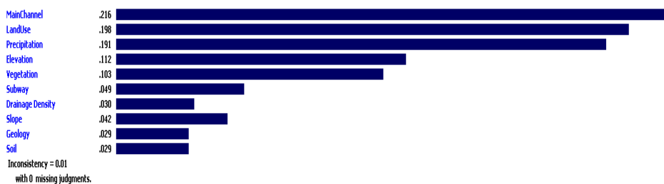
شکل (۳). وزن‌های بدست آمده برای معیارها و میزان ضریب ناسازگاری (منبع: نگارندگان)
