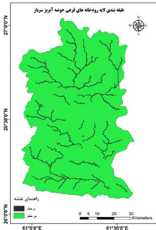
شکل (۱۴). طبقه بندی لایه رودخانه فرعی از نظر پتانسیل سیل خیزی (منبع: نگارندگان)
