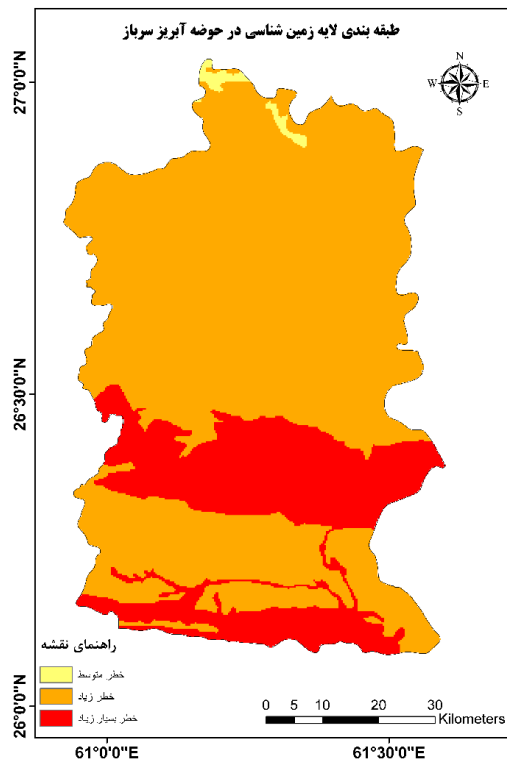
شکل (۵). طبقه‌بندی لایه زمین‌شناسی حوضه آبریز سرپاز بر حسب پتانسیل سیل خیزی (منبع: نگارندگان)
