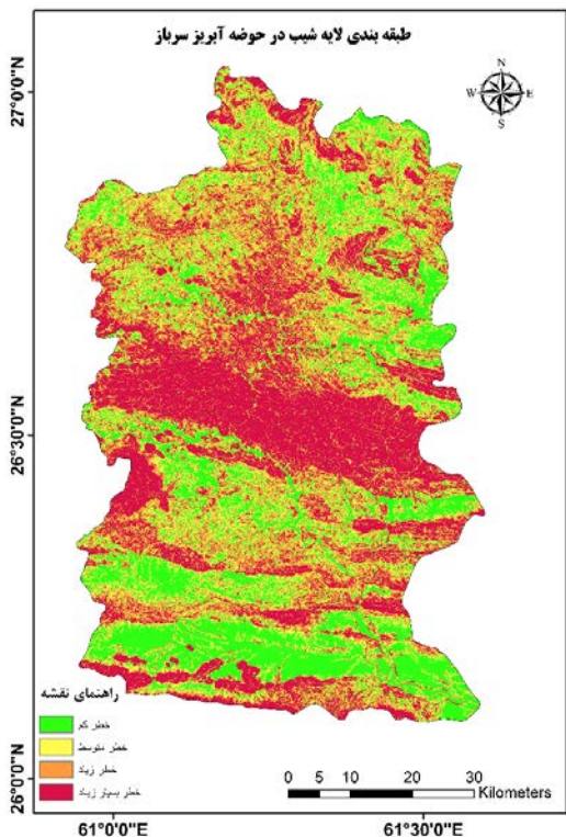
شکل (۶). طبقه‌بندی لایه شیب حوضه آبریز سرپاز بر حسب پتانسیل سیل خیزی (منبع: نگارندگان)
