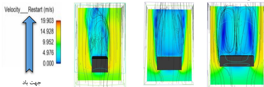
نسبت طول به عرض ۳ به ۱ نسبت طول به عرض ۲ به ۱ نسبت طول به عرض ۱ به ۱ شکل ۴: مطالعه‌ی سایه‌ی باد از طریق شبیه‌سازی مکعب با ابعاد مختلف در برابر باد
