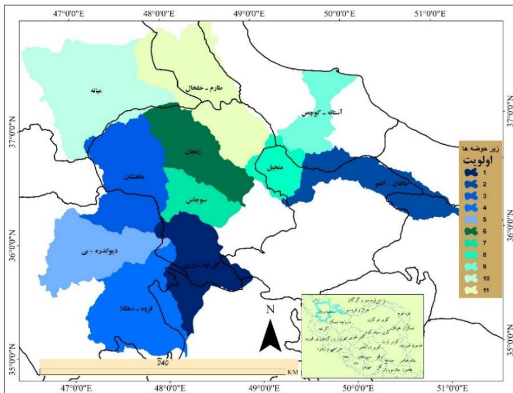
شکل ۴: نقشه‌ی اولویت بندی نهایی زیرحوضه‌ها با استفاده از تلفیق نرخ فرسایندگی، پوشش گیاهی و مورفومتری
