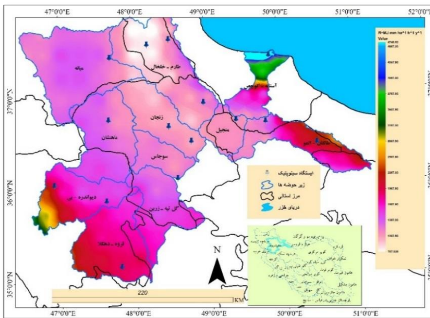
شکل ۲: نقشه‌ی فرساینده‌گی حوضه‌ی آبریز سفیدرود بزرگ بر اساس داده‌های بارش TRMM
