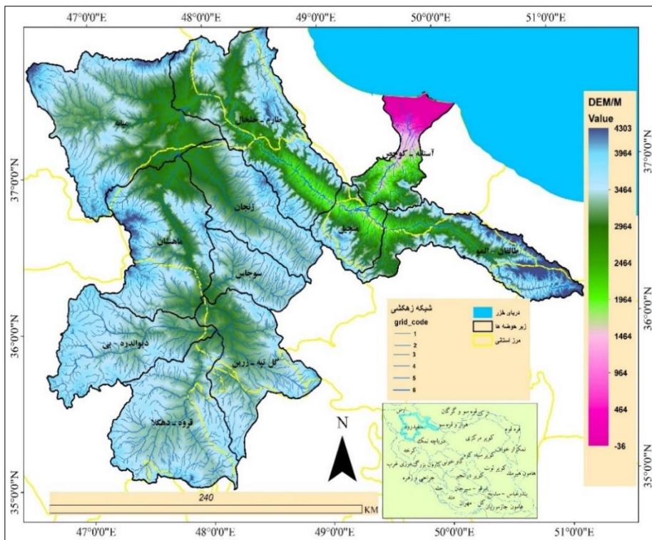
شکل ۱: موقعیت حوضه‌ی آبریز سفیدرود در میان حوضه‌های آبریز کشور
