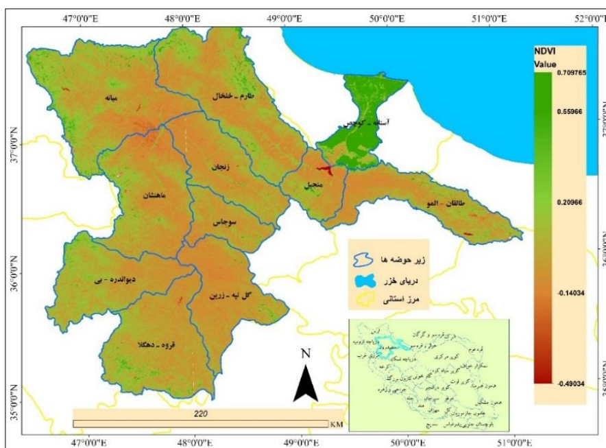
شکل ۳: نقشه‌ی پوشش گیاهی حوضه‌ی آبریز قزل اوزن-سفیدرود بزرگ بر اساس شاخص NDVI و تصاویر MODIS
