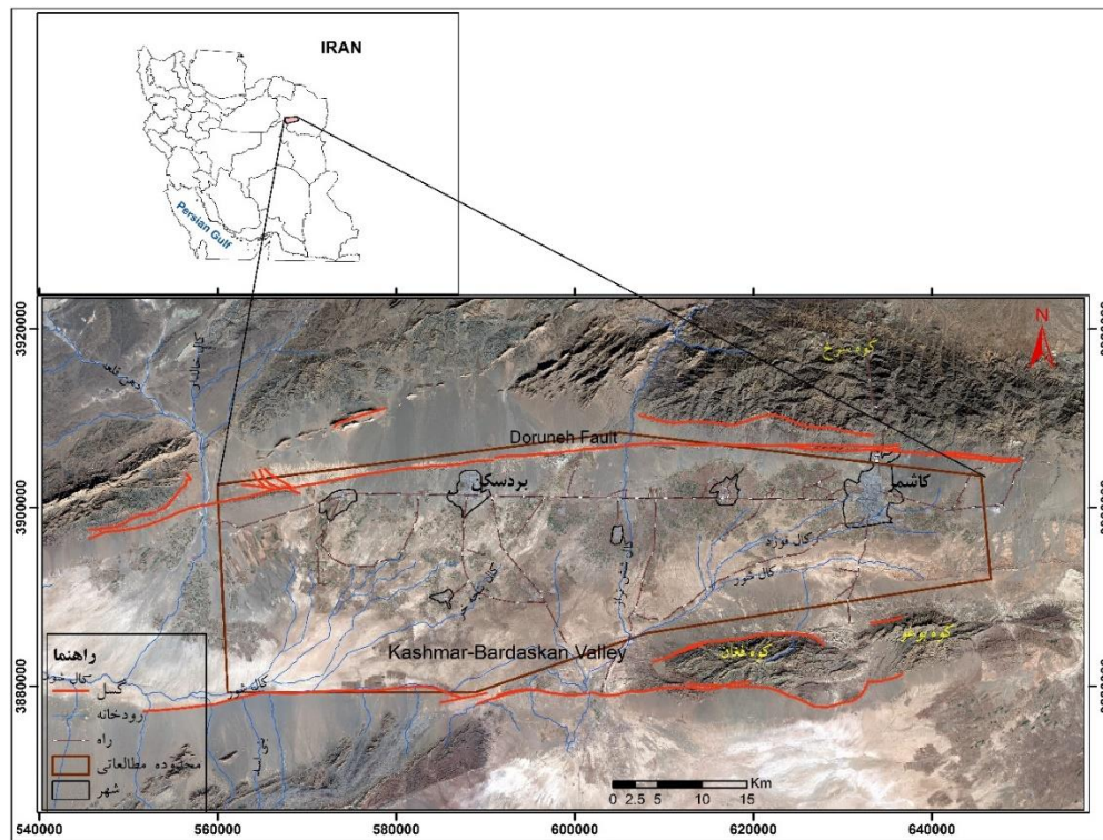
شکل ۱: موقعیت محدوده‌ی مطالعاتی دشت کاشمر-بردسکن بر روی تصویر ماهواره‌ی Sentinel-2
