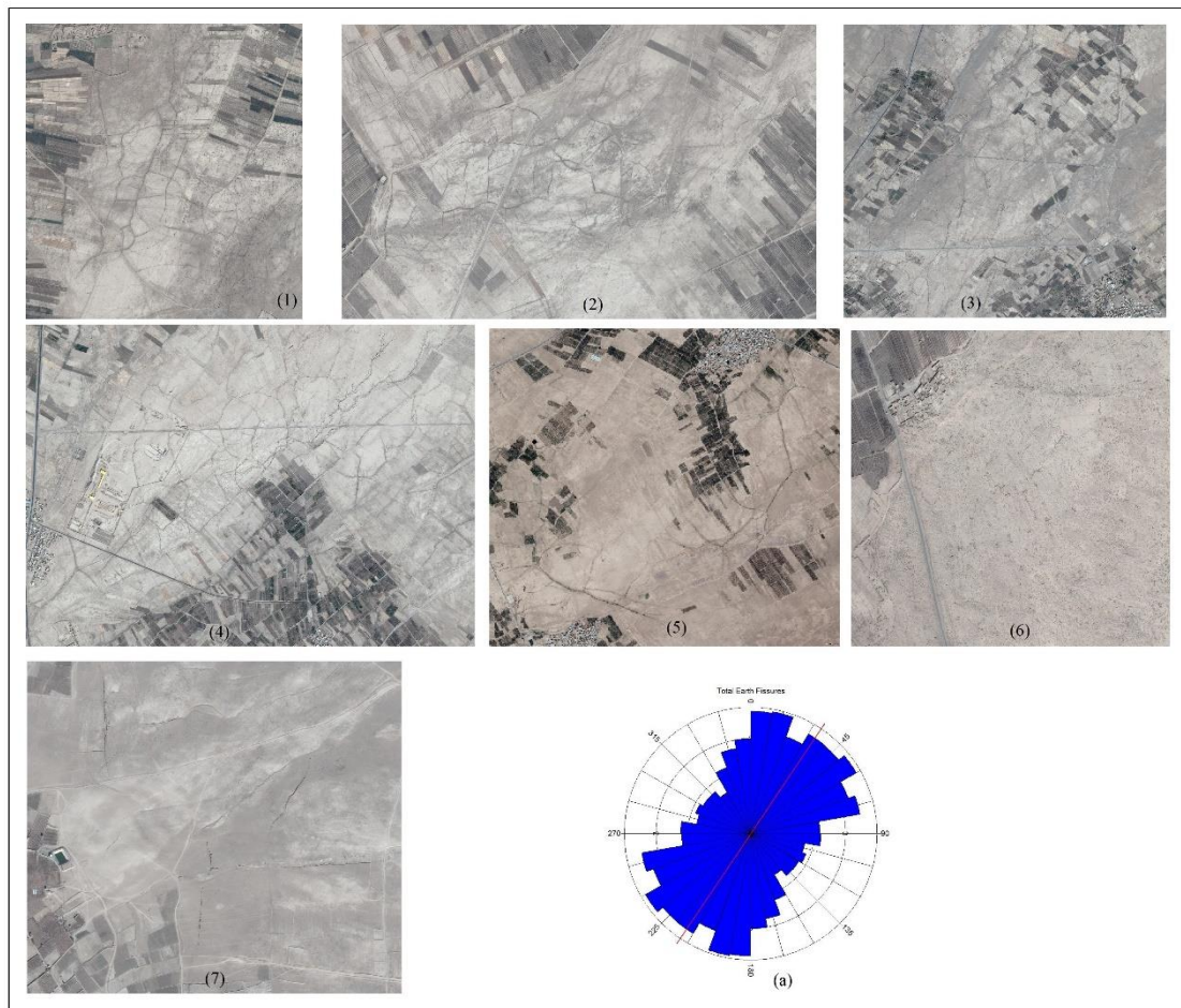
شکل ۷: الگوی درز و شکاف‌ها در روستاهای؛ (۱) شرق شریعت‌آباد (۲) جنوب زمان‌آباد (۳) شمال غرب زیرک‌آباد (۴) شمال شرق کلاته نو (۵) جنوب کوشه (۶) چراغ چین (۶) کلاته شادی (a) دیاگرام گل‌سرخ‌ی درز و شکاف‌ها در دشت کاشمر-بردسکن
