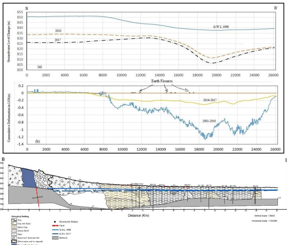
شکل ۱۱: پروفیل B-B' (a) تغییرات سطح آب زیرزمینی و (b) تغییرات فرونشست زمین و محل تشکیل درز و شکاف‌ها (c) نیمرخ زمین‌شناسی در راستای پروفیل
