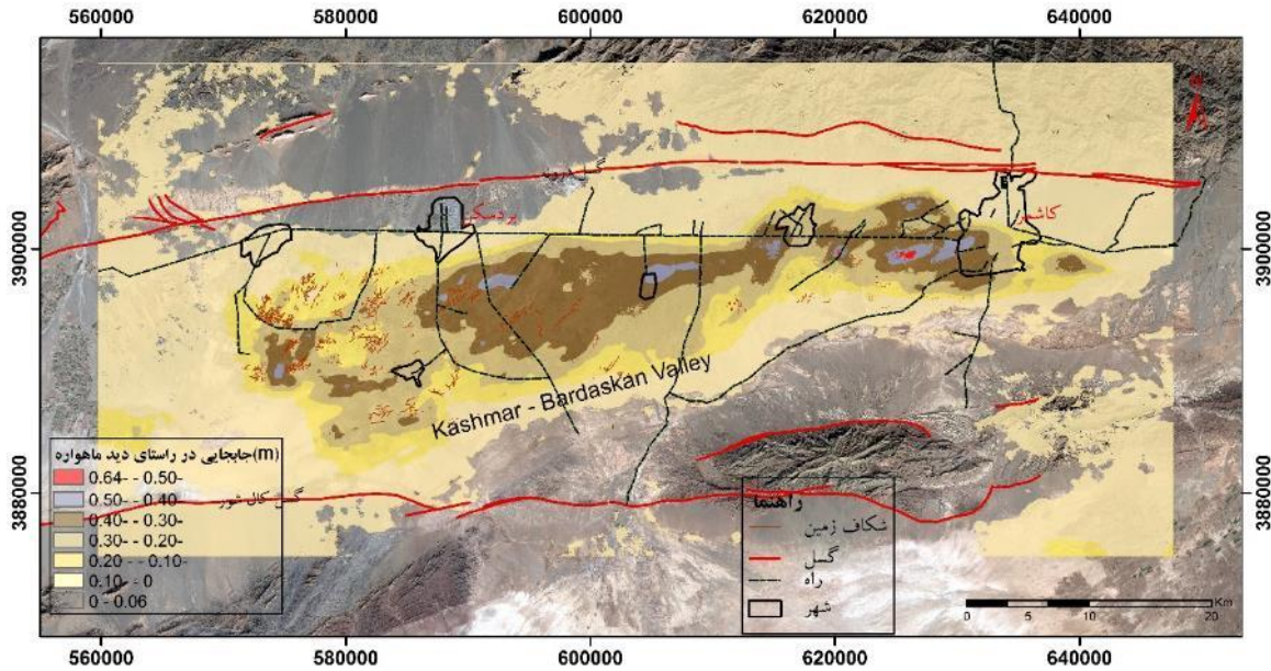
شکل ۴: فرونشست تجمعی در راستای دید ماهواره با استفاده از تصاویر Sentinel-1 در بازه زمانی ۲۰۱۷-۲۰۱۴ در دشت کاشمر-بردسکن
