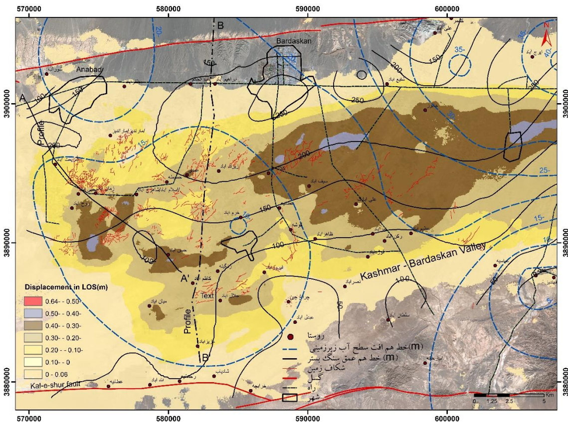
شکل ۹: ارتباط درز و شکاف‌ها با فرونشست و عمق سنگ بستر در مرکز و غرب دشت کاشمر-بردسکن طی سال‌های ۲۰۱۷-۲۰۱۴
