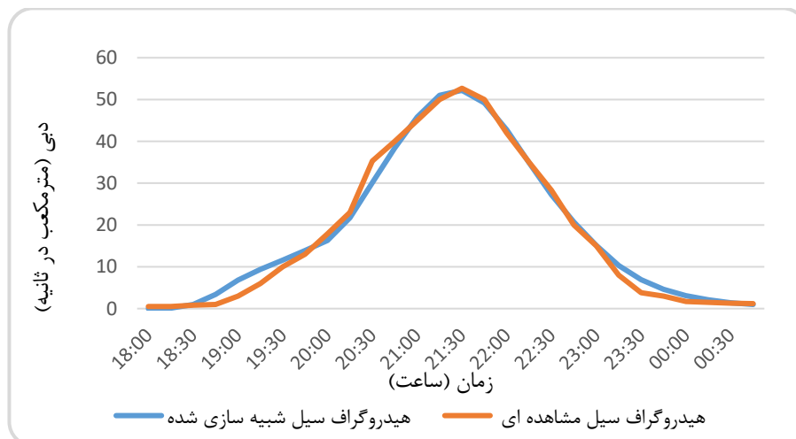
شکل ۵: هیدروگراف سیل مشاهده‌ای و شبیه‌سازی‌شده حوضه‌ی آبخیز در مرحله‌ی واسنجی
