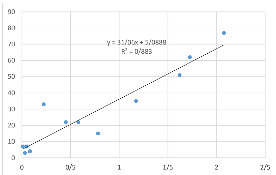
شکل ۹: نمودار ضریب همبستگی بین میزان فرونشست زمین و افت سطح آب چاه‌ها
