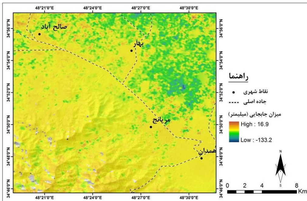
شکل ۶: نقشه میزان جابجایی منطقه از تاریخ ۲۰۱۶/۰۱/۱۱ تا ۲۰۱۷/۱۲/۱۹
